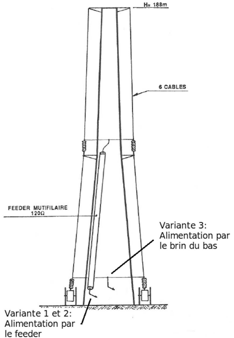
Schéma électrique du grand pylône, avec les variantes d'alimentation essayées.
