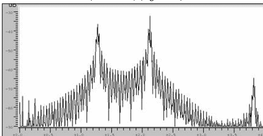
SIGNAL RTTY SHIFT LARGE (850 Hertz) (signal reçu entaché d'un bruit important)
