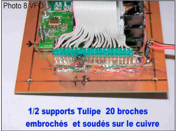
VFO PA0KLT sur plaque époxy cuivrée 100 X 160 mm
