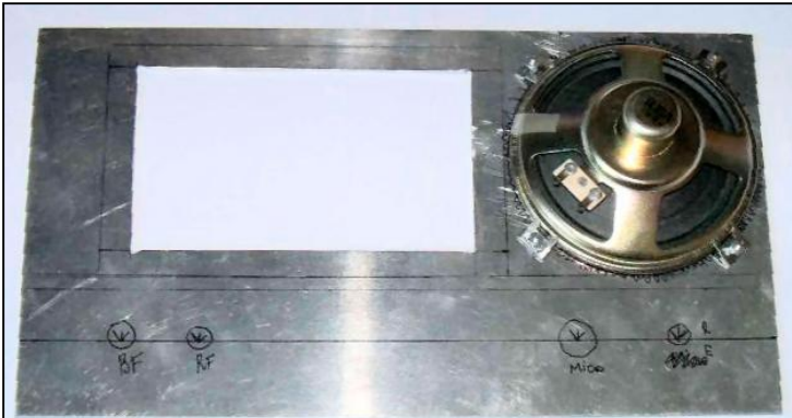
Façade en Alu e= 1,5mm 165 x 300 mm
