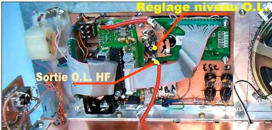
Le câble coaxial miniature (rouge) d'injection de l'OL passe au travers du châssis, le générateur BINGO SSB est en dessous
