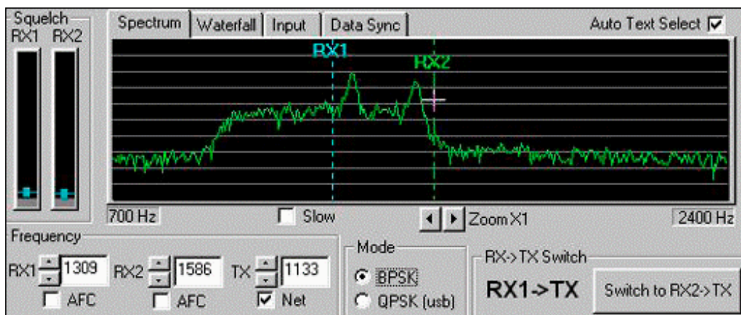
Largeur de bande de 500 Hz
