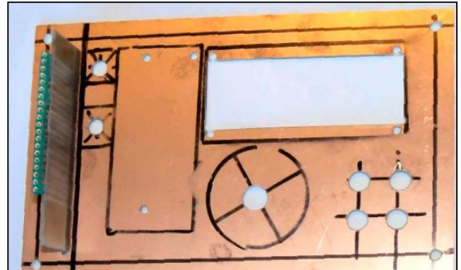
VFO implanté sur époxy simple face
