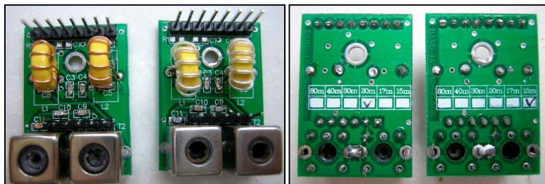
Platines embrochables bande
