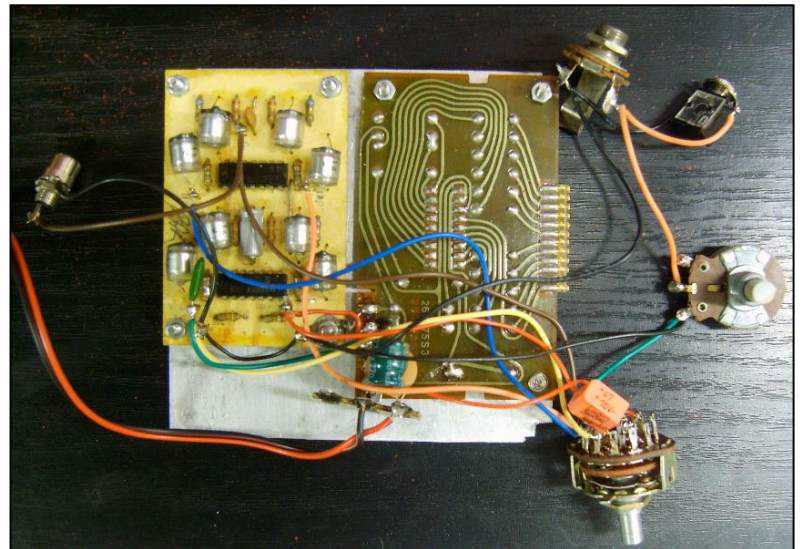
Les deux circuits montés sur une plaque d'aluminium qui sera glissée dans les rainures du boîtier en alu extrudé..
