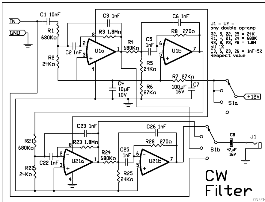
Notre filtre CW à quatre pôles. Ci-dessous, le livre de Vecronics
