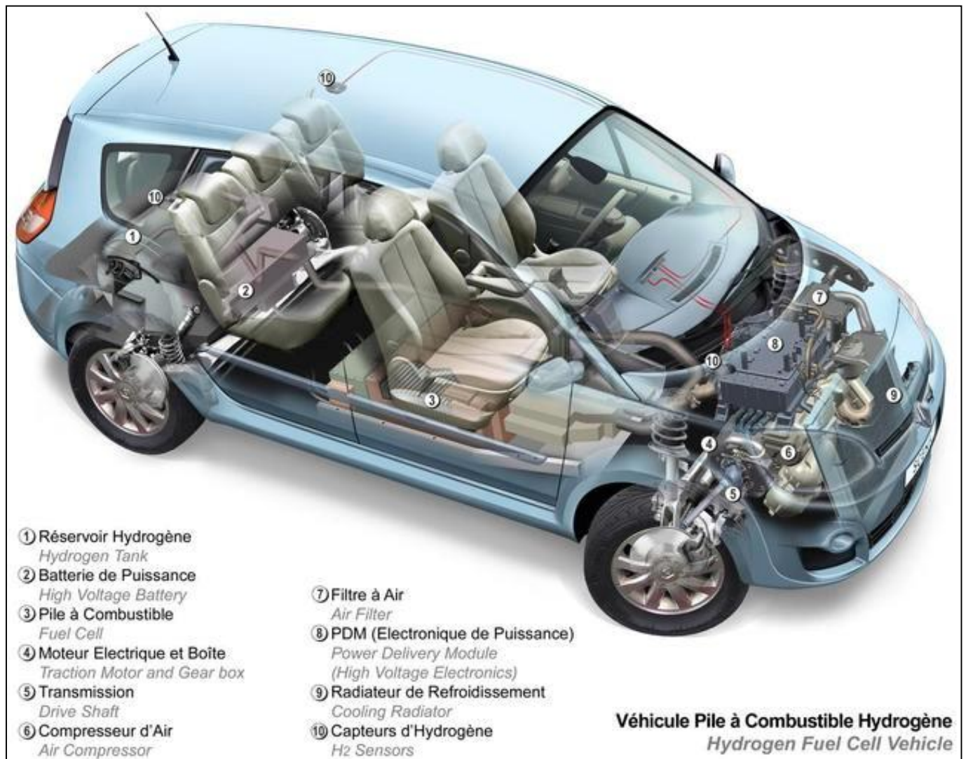
La Renault Scenic ZEV H2 (Renault - Nissan) utilisant une pile à combustible hydrogène. Le problème subsiste le volume des équipements par rapport à l'espace disponible.
