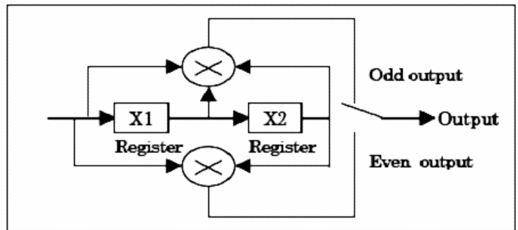
Figure 3: Schéma de l'algorithme de convolution [1]
