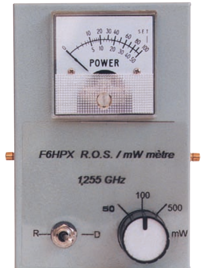
Figure 8 : ROS Rapport d'Ondes Stationnaires (tension ou courant).
