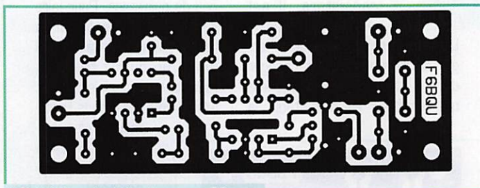
Circuit imprimé du récepteur 80m à quartz.
