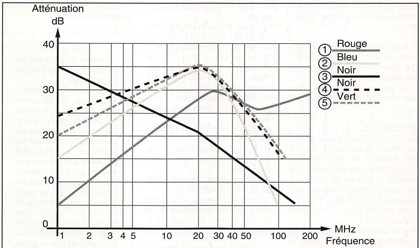
Figures 5. Atténuation apportée par quelques inductances d'arrêt en fonction de la fréquence.
