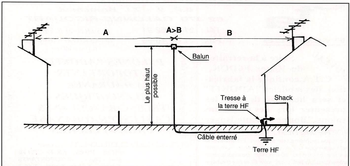
Figure 1. Emplacement d'une antenne (voir le texte).
