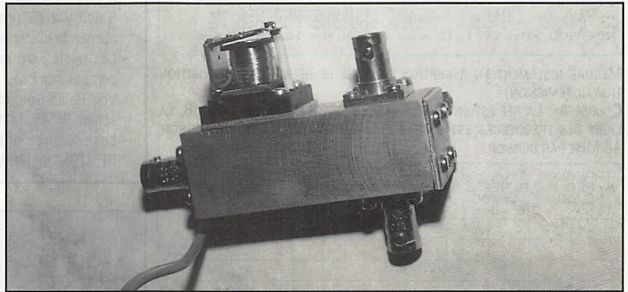
Relais coaxial 50 Ω équipé fiche BNC. Observez le montage de la bobine de relais automobile et le système de transfert de mouvement réalisé avec l'aide d'un batonnet de céramique récupéré sur un vieux fer à souder. * La bobine est surélevée à l'aide d'un morceau d'epoxy.
