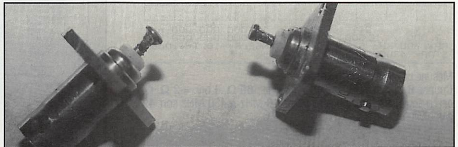
Relais coaxial 50 Ω. Détail de montage (soudure) des contacts sur les broches des BNC. Voir plan pour dimensions.
