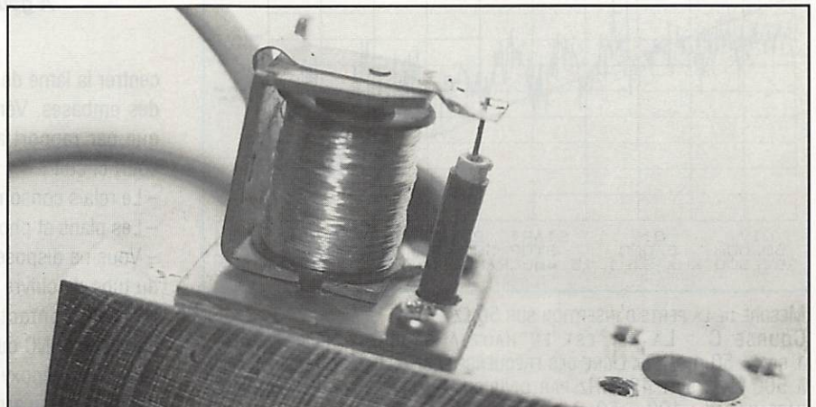
Relais coaxial 50 Ω. Détail de la bobine de commande.
