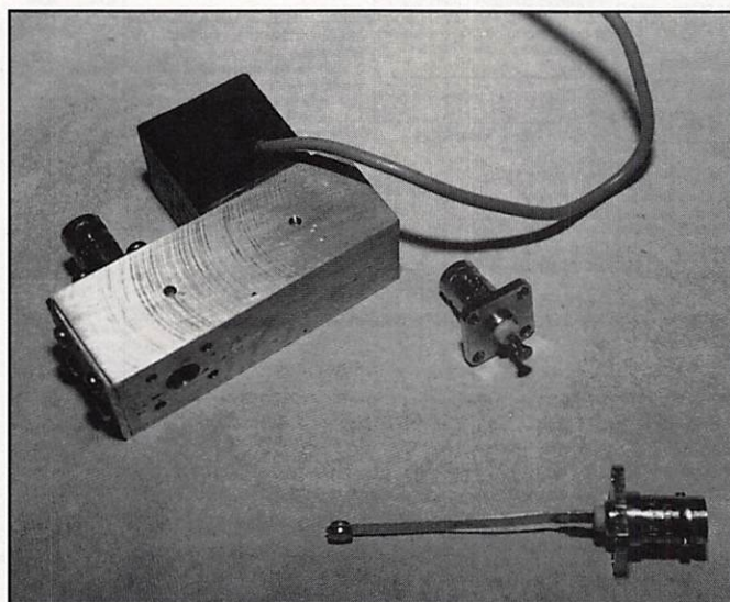
Relais coaxial 50 Ω partiellement démonté pour présenter la BNC équipée d'une pastille de contact et l'autre de la lame de contact.
