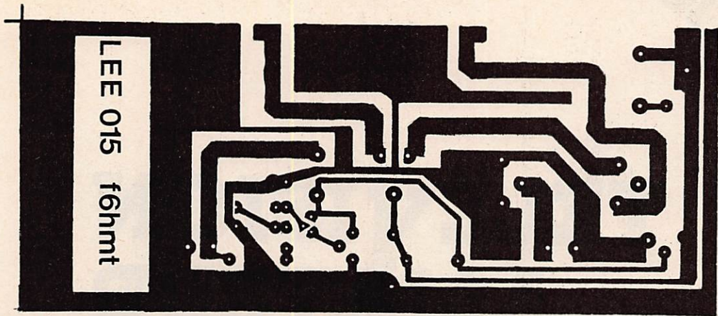
Commutation dessous
