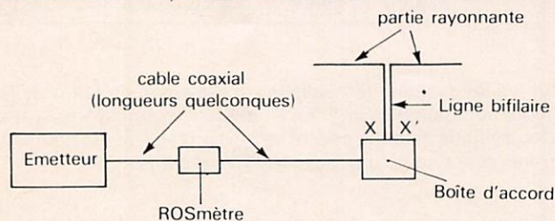
Figure IV.2.5d. - Avec les émetteurs modernes, il est nécessaire de passer par une boîte d'accord avant d'attaquer la ligne bifilaire. Le ROS mètre placé sur la ligne coaxiale permet de vérifier la qualité du réglage.
