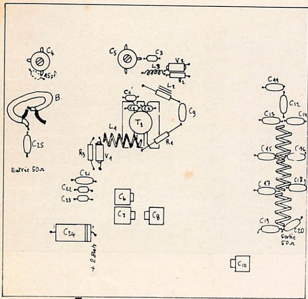
IMPLANTATION ECHELLE 1/2
