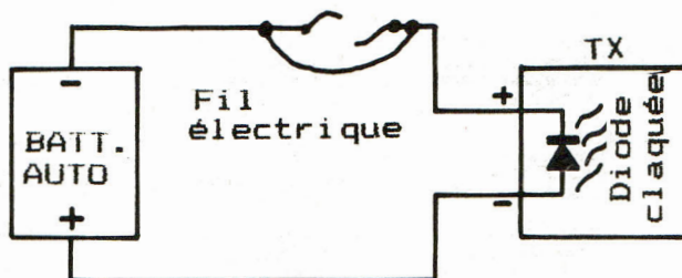
Fusible remplacé par un fil électrique: destruction de la diode qui devient un court-circuit permanent.
