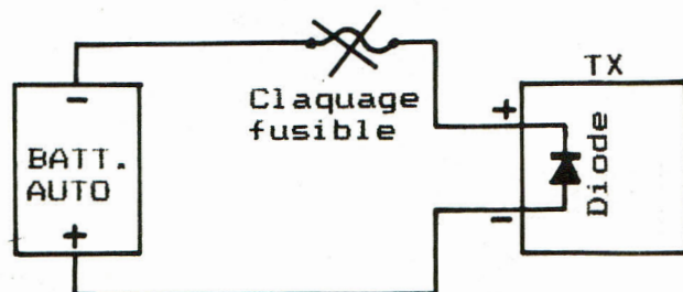
Fonctionnement de la protection à diode.
